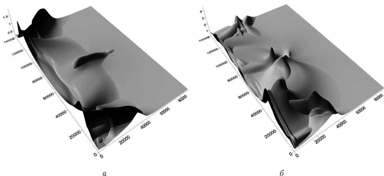
Рис. 4. Картины “свечения” — максимальных значений амплитуд за все время расчета: a — в случае оползня, стартовавшего по центру желоба, b — с его края
