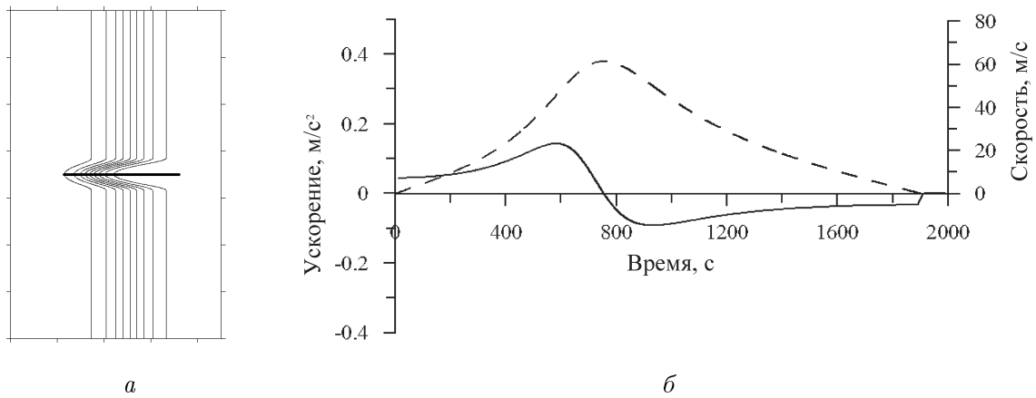
Рис. 2. Характеристики движения центра масс оползня, стартовавшего по центру желоба: a — траектория движения (жирная линия) на фоне изолиний глубин; b — соответствующие скорости (штрих) и ускорение (сплошная линия) вдоль оси Ox
