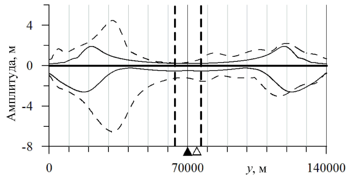
Рис. 5. Распределения максимальных и минимальных высот волн, рассчитанные в береговых точках: сплошные линии соответствуют оползнию, стартовавшему по центру желоба, штриховые — с его края. Треугольниками отмечены начальные y -координаты центров масс: сплошной соответствует первому случаю, контурный — второму. Вертикальные штриховые линии указывают границы желоба
