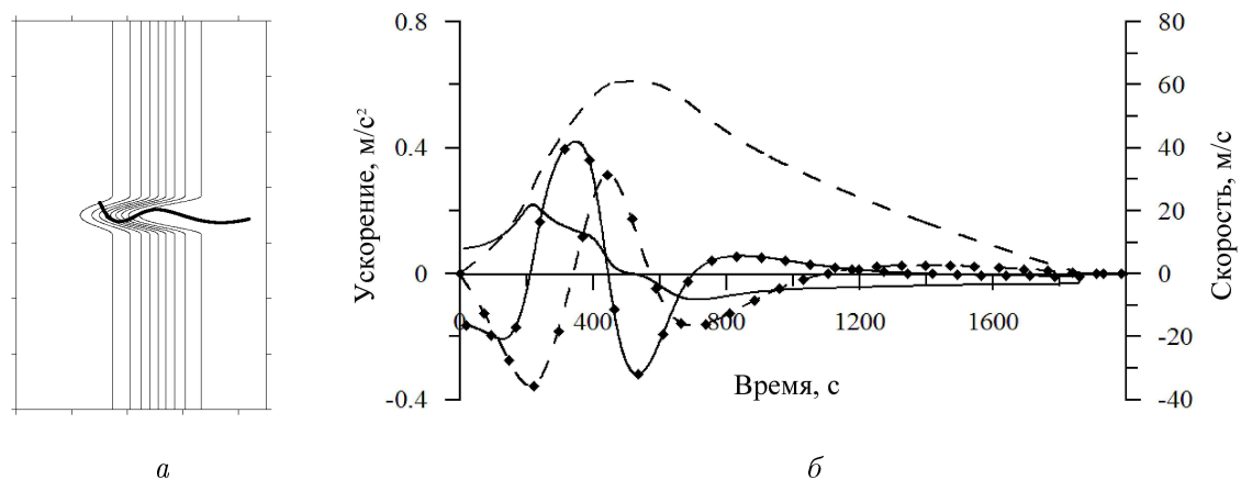
Рис. 3. Характеристики движения центра масс оползня, стартовавшего с края желоба: a — траектория движения (жирная линия) на фоне изолиний глубин; b — соответствующие скорости (штрих) и ускорения (сплошные линии); кривые без маркеров соответствуют значениям вдоль оси Ox , с маркерами — Oy
